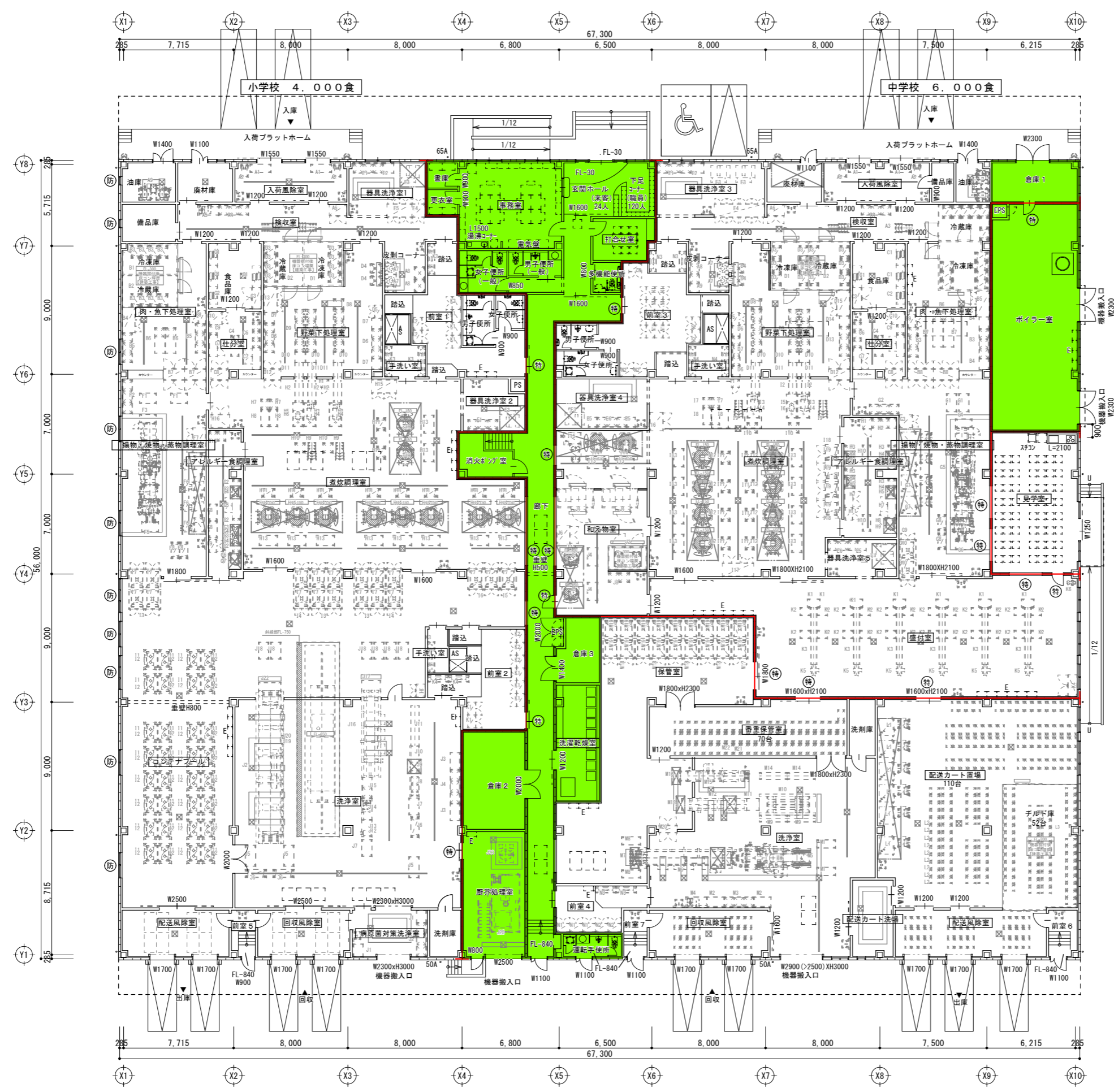
1階平面図・厨房機器配置図
