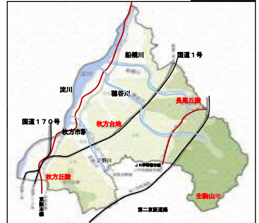
地形図
